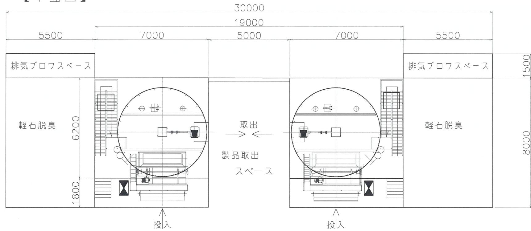
【平面図】
