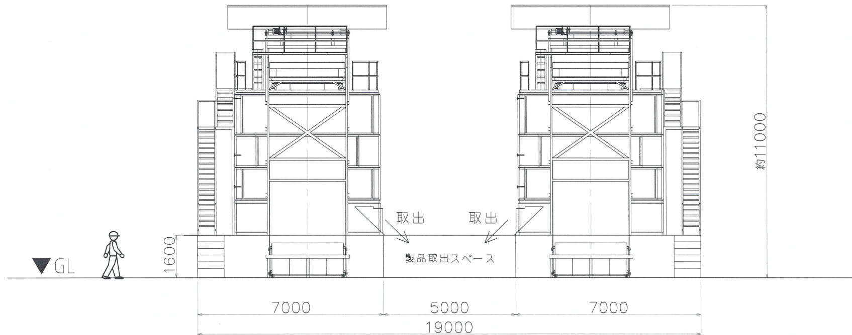
【正面図】
